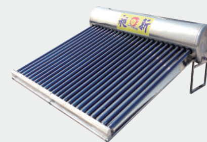
CSB-3524 適用人數6-9人
